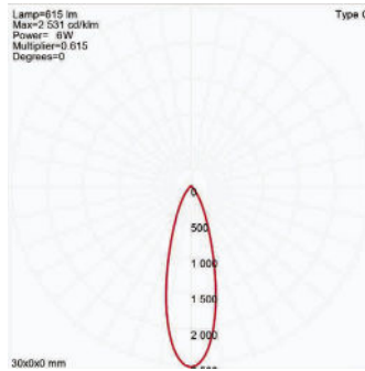
45° FWHM TIR
